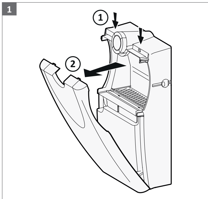
Gerät ausschalten und Frontblende öffnen Switch off the unit and open front panel
