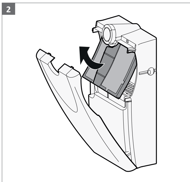
Filterrahmen und Filter entnehmen Remove filter frame and filter
