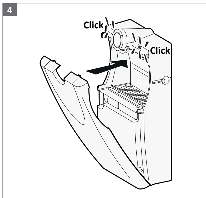
Frontblende schließen Close front panel
