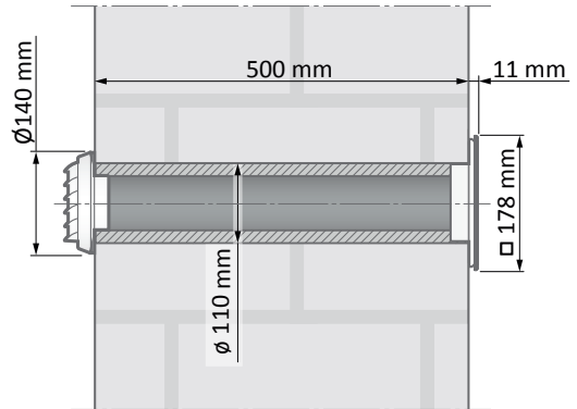
AEROTUBE DD 110 mit Innenblende E18 und Wettschutzgitter
