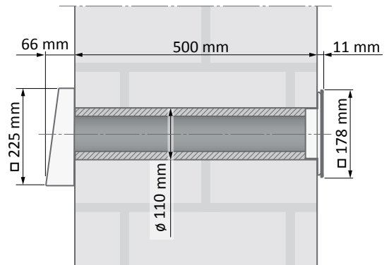
AEROTUBE DD 110 mit Innenblende E18 und Wettschutzhaube
